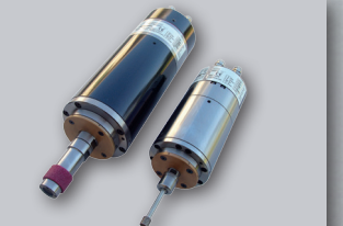
Taşlama mili
