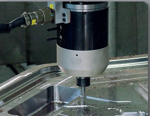
Yardımcı mili
